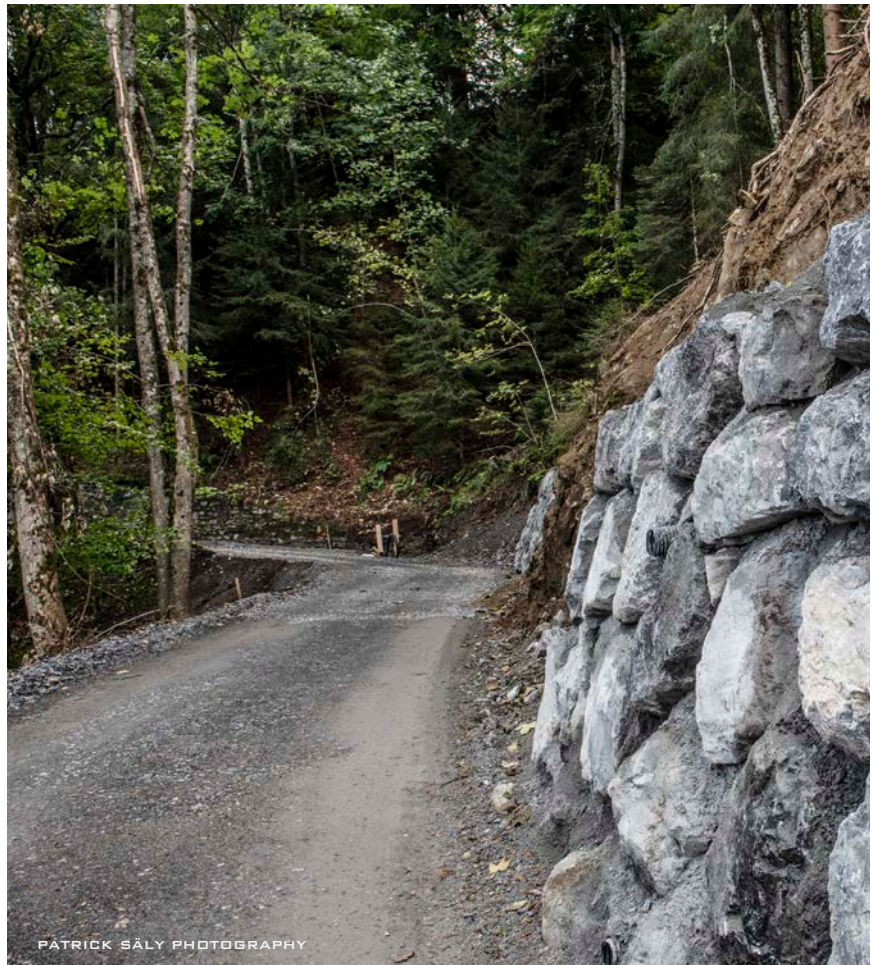
Hangsicherung bei der Zufahrtsstraße Bitschweil
